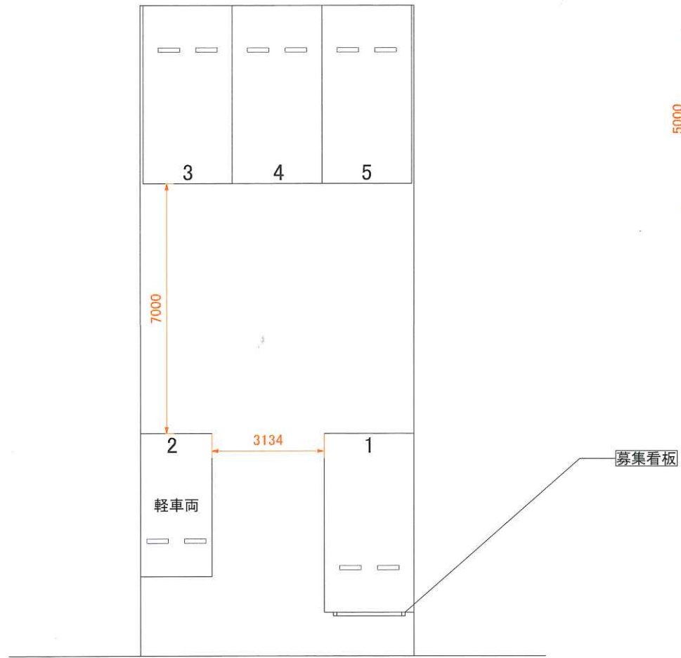
車室寸法
