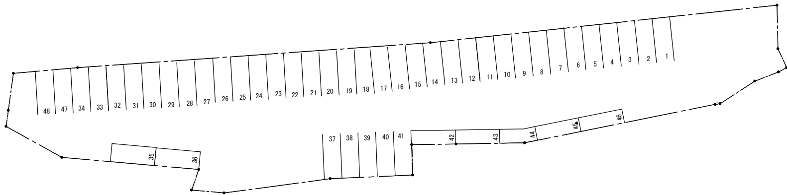
新宮駐車場 平面図 S=1/300
